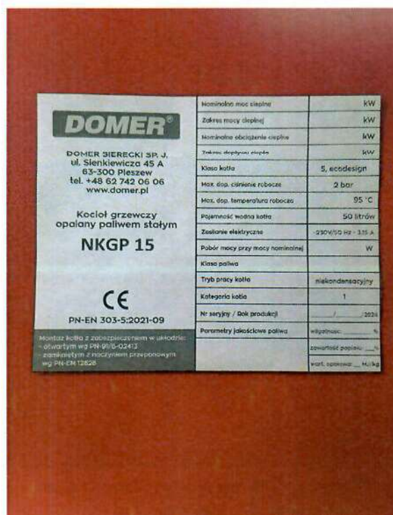
Rysunek 17 Tabliczka znamionowa
